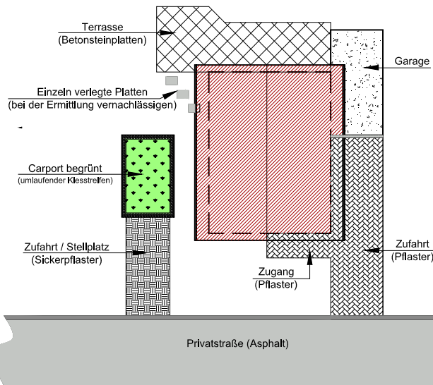
Draufsicht (Vogelperspektive)
